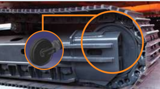
Resorte de orugas y rueda guía integrados
